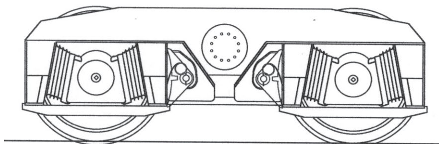
Boggie SEAG med Megi-fjädring. Axelavstånd i boggie 1700 mm
