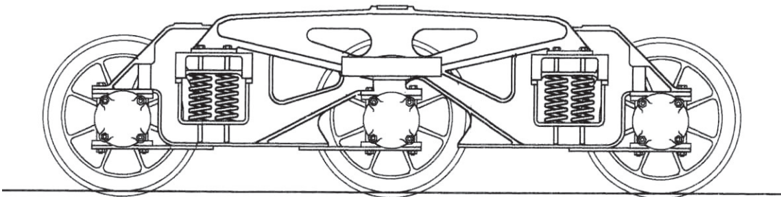
Treaxlig boggie till transformatorvagn litt Q19 nr 23010, 34619. Axelavstånd i boggie 3000 mm (6000 mm över ytteraxlar)
