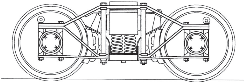
SJ standardboggie mod 46A av Diamondtyp. Återfanns under vagnar litt lbr nr 102000-102100 m.fl. Axelavstånd i boggie 1680 mm.
