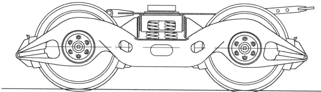
Henricotboggie, en boggietypp som endast undantagsvis har använts under svenska godsvagnar. Axelavstånd i boggie 1800 mm.
