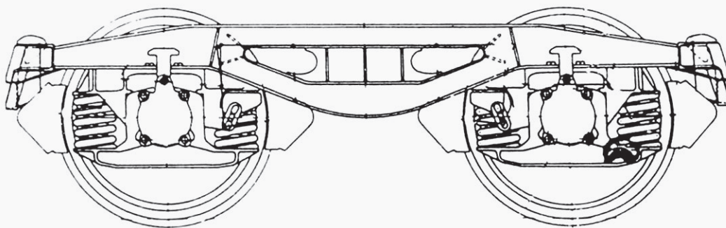
Standardboggie för godsvagnar med Y25 (ORE standardboggie sedam 1967). Axelavstånd i boggie 1900 mm.
