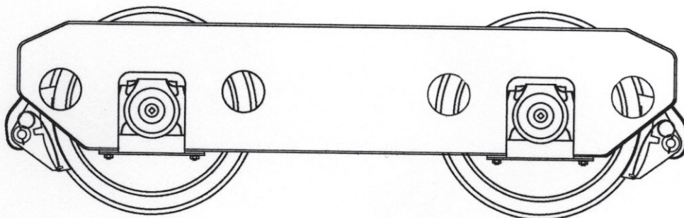
Boggie för provmalmvagn nr 106748 variant 1 (ASJ Falun). Axelavstånd i boggie 1800 mm
