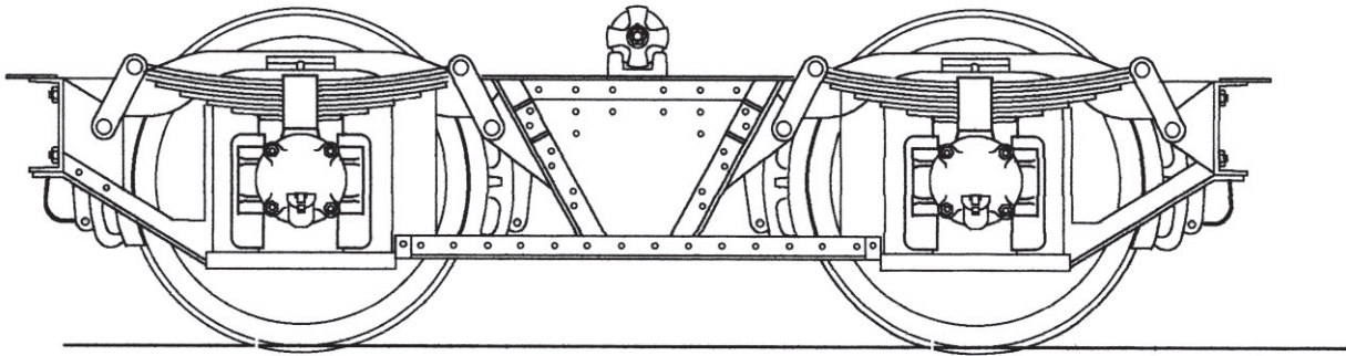
Boggie mod 34 i nitat utförande för öppna godsbyggvagnar litt Ob. Axelavstånd i boggie 2000 mm.
