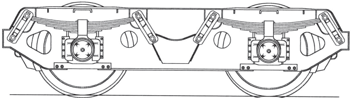
SJ Standardboggie med G56 (UIC standardboggie för godsvagnar). Axelavstånd i boggie 2000 mm.
