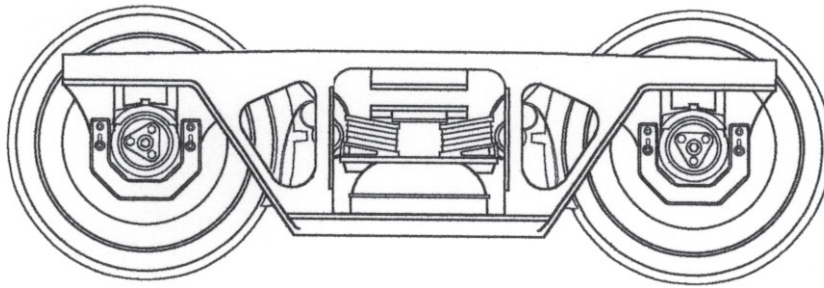
Boggie modell G 871 - ASEA-boggien, provades i en av SSAB:s stålämnesvagnar, axelavstånd i boggie 1800 mm. Boggierna var misslyckad och togs tidigt ur tjänst.
