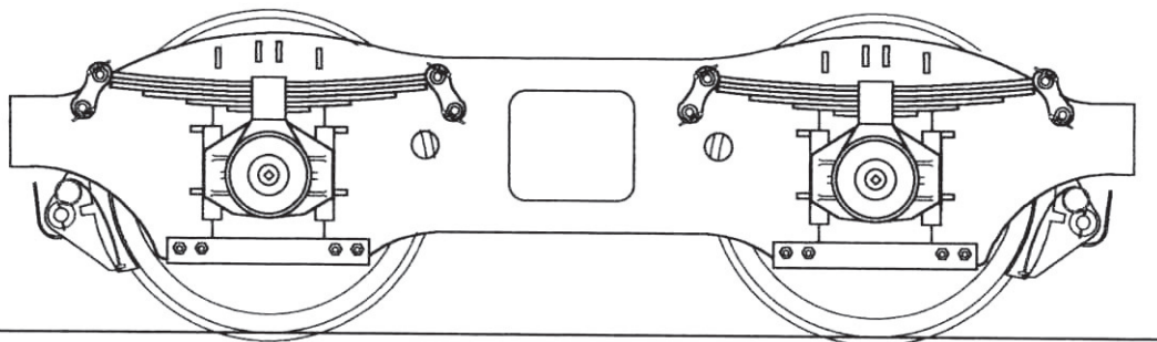
Boggie för korta tankvagnar litt Q12b. Utgöres av tenderboggierna från DR och byggdes in i tankvagnar levererade av Raxwerk i Österrike. Boggierna och vagnarna var nybyggda med användning av kvarblivet material. Axelavstånd i boggie 1800 mm.
