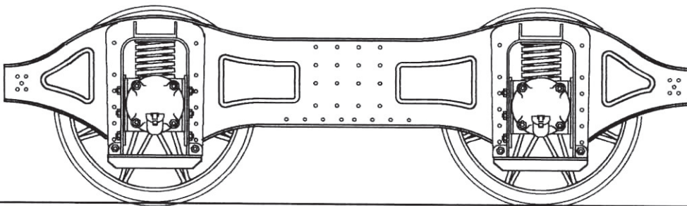
Boggie av Foxtyp för öppna godsvagnar med höga väggar litt lb med nr 29895-29944. Axelavstånd i boggie 1800 mm.
