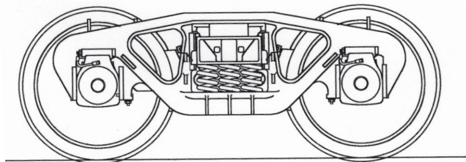
SJ Standardboggie mod G 673 (för malmvagnar), fabrikat Henricot. Axelavstånd i boggie 1800 mm
