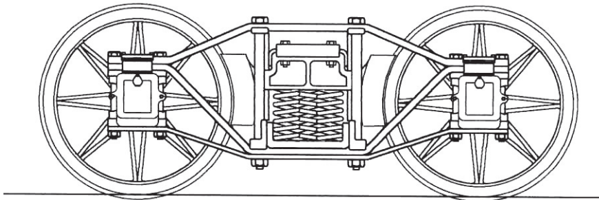
Boggie för malmvagn litt Mo nr 15317-15336. Vagnarna såldes sedermera till LKAB. Axelavstånd i boggie 1630 mm.
