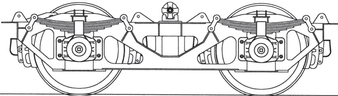
Boggie mod 34 i svetsat utförande för öppna godsbyggvagnar litt Ob. Axelavstånd i boggie 2000 mm.
