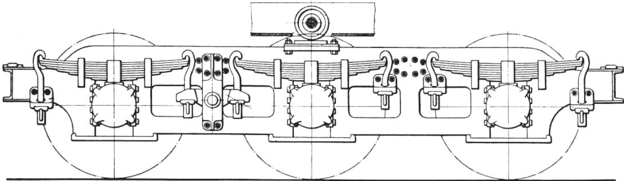
Treaxlig boggie för vagnar litt So nr 22759 - 22760 (fd litt Sd) m.fl. Axelavstånd mellan boggieaxlar 2600 mm (5200 mm över ytteraxlar).
