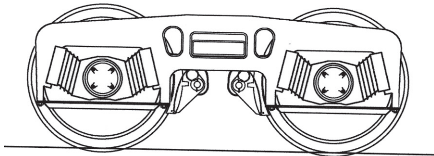
Boggie för provmalmvagn nr 106758-759, SJ Maskinbyrån mod G 65, tillverkare Henricot i gjutet utförande. Axelavstånd i boggie 1500 mm
