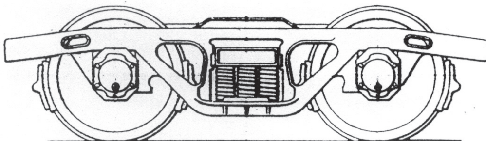
Boggie för provmalmvagn litt Mb nr 106746. Axelavstånd i boggie 1800 mm.
