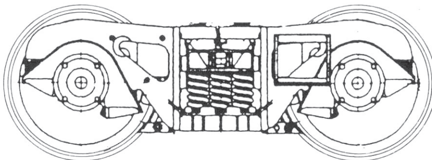
LKAB Malmvagnsboggie av Scheffeltyp för Sydafrikavagnarna. Axelavstånd i boggie 1800 mm.
