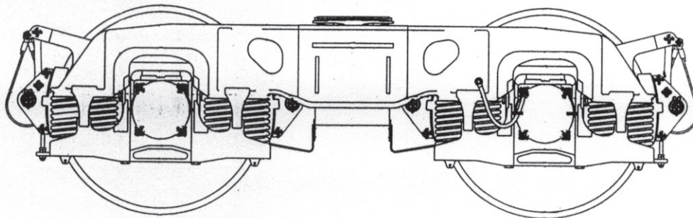
Boggie från NACU technologies (numera Probotec) för 30 tons axellast, mod G 981. Aterfinns under en del stålämnesvagnar. Axelavstånd i boggie 1700 mm.
