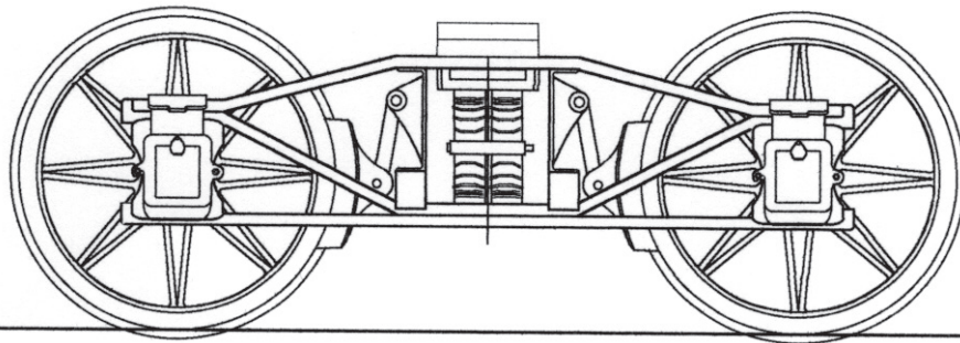
Skåne-Hallands Järnvägars (SHJ) boggie till öppna godsvagnar litt No. Axelavstånd i boggie 1850 mm.
