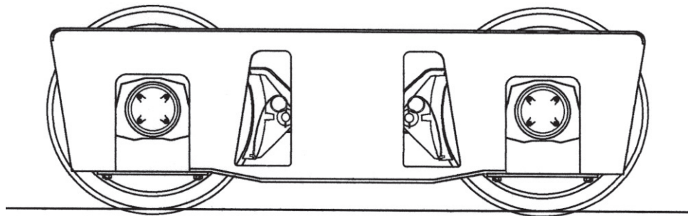
Boggie för provmalmvagn nr 106748 variant 3. Axelavstånd 1800 mm
