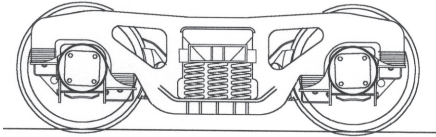
Scheffel HS radial (LKAB Uanoo), axelavstånd i boggie 1800 mm.
