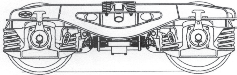
Standardboggie mod Y 31. Axelavstånd i boggie 1800 mm.
