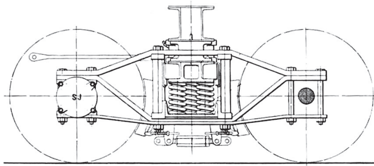
Boggie av typ Diamond för tidigare varianter av transformatorvagn litt Q1 nr 23741. Axelavstånd i boggie 1500 mm.
