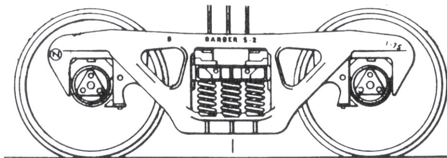
Boggie för provmalmvagn nr 106745. Axelavstånd i boggie 1800 mm.
