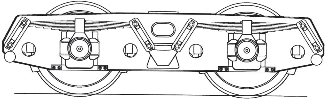
SJ standardboggie mod G70 med kortare axelavstånd om 1800 mm.
