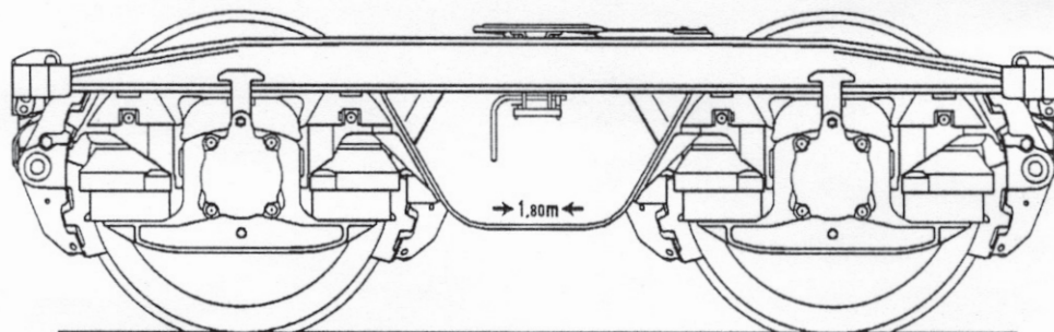
Talbot godsvagnsboggie typ DRRS-25. Axelavstånd i boggie 1800 mm. Förekommer i Sverige under ett antal av Nordwaggons vagnar.
