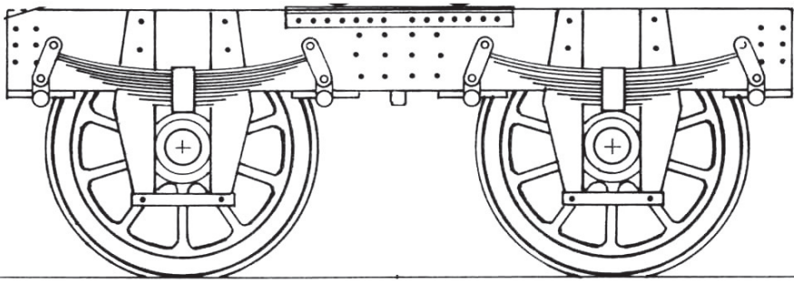
Boggie för kanonvagn litt Q1 nr 4061, 5649-5650. Axelavstånd i boggien 1575 mm.
