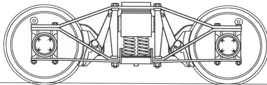
Boggie av typ Diamond för tankboggievagnar. Axelavstånd i boggie 2000 mm.
