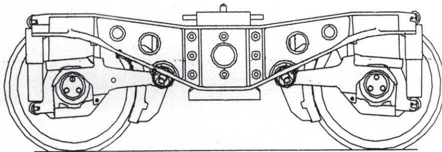
Standardboggie typ TF25. Axelavstånd i boggie 2000 mm. Har ännu ej använts i Sverige
