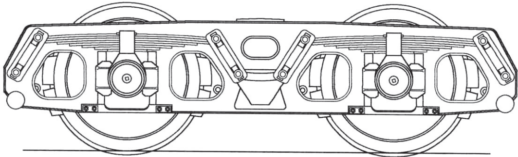
SJ standardboggie mod G66 med kortare axelavstånd om 1800 mm.
